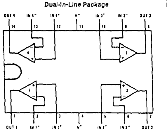
TL/H/5647-1
